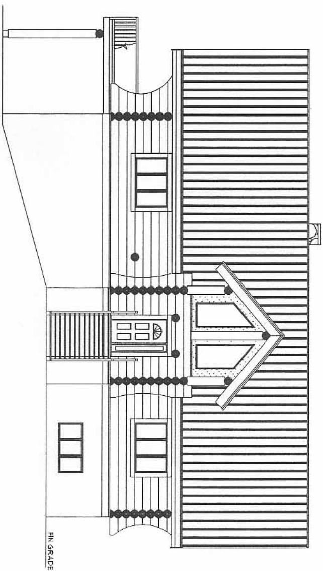
RIGHT ELEVATION
